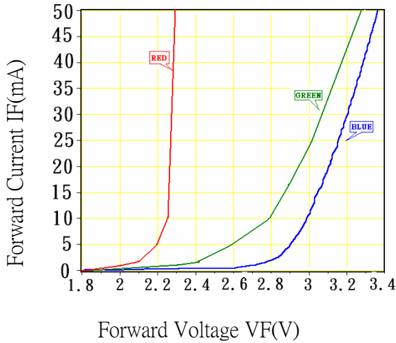
Fig.1 IF-VF(Ta=25°C)
