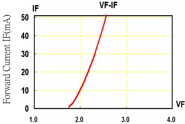
Fig.1 IF-VF(Ta=25°C)
